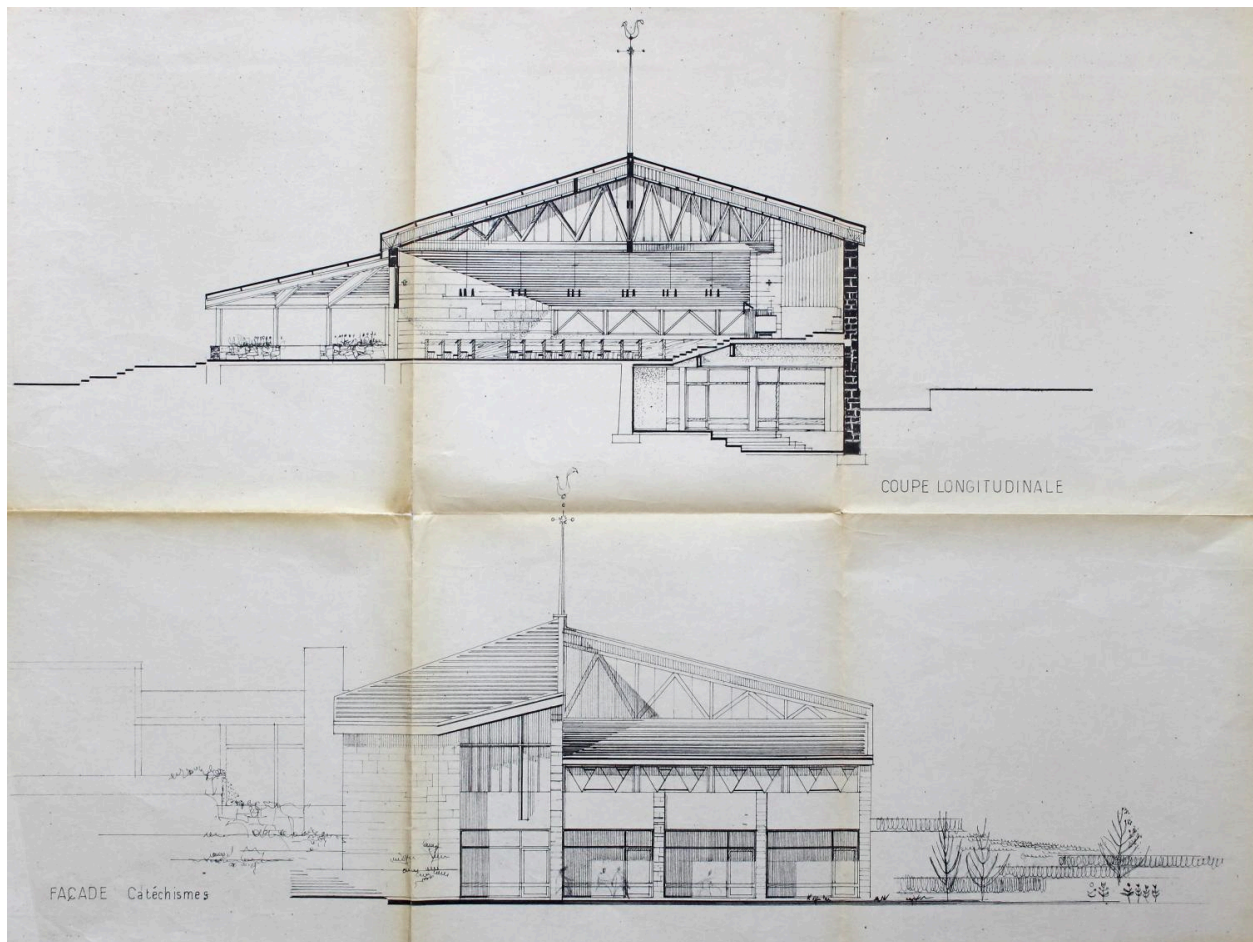
Brioude, chapelle de la Borie Darles, « coupe longitudinale et façade catéchisme », avant-projet non daté (vers juin 1964), Guy Bion architecte, Archives de la paroisse Saint-Julien de Brioude.
