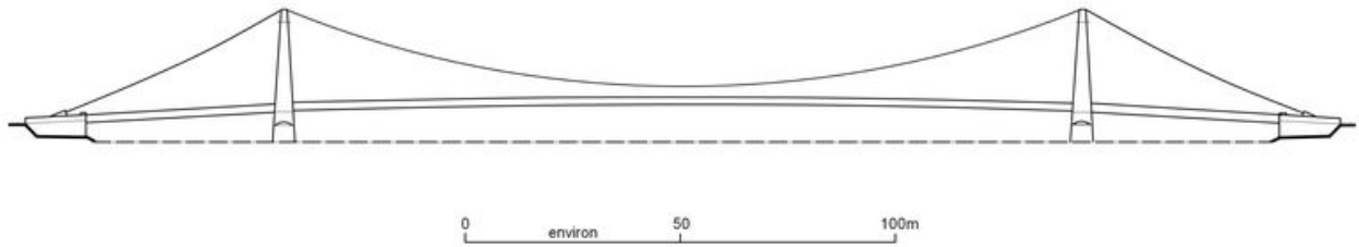
Elévation (relevé schématique)
