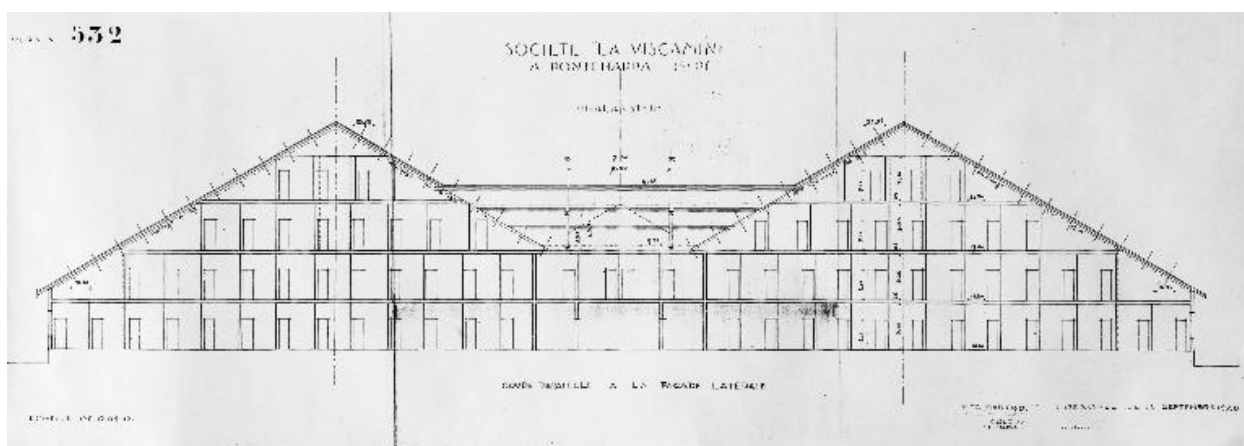
Phalanstère. Coupe parallèle à la façade latérale (1928)
