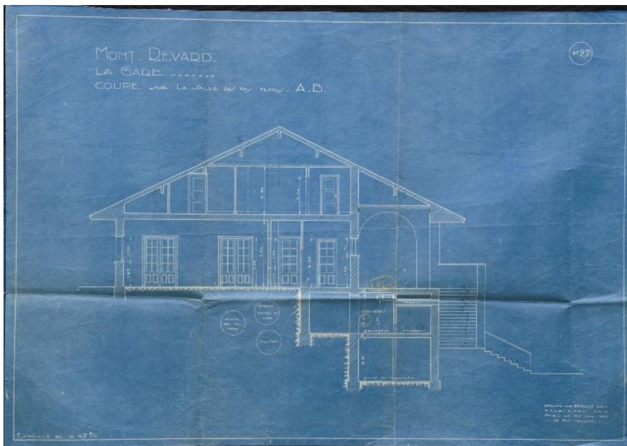
Coupe sur la salle des pas perdus, 1924
