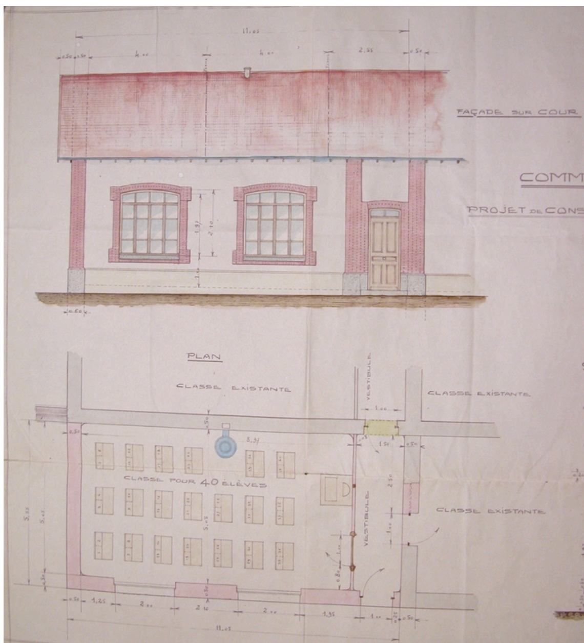
Commune de Savignoux. Projet de construction d'une classe enfantine. Façade sur cour. Plan. 1928.
