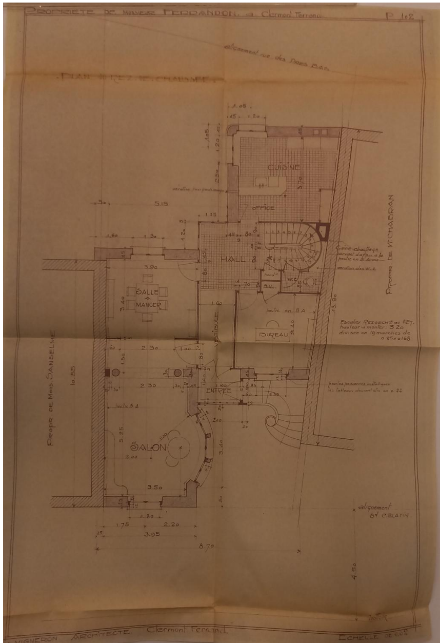
Plan du rez-de-chaussée
