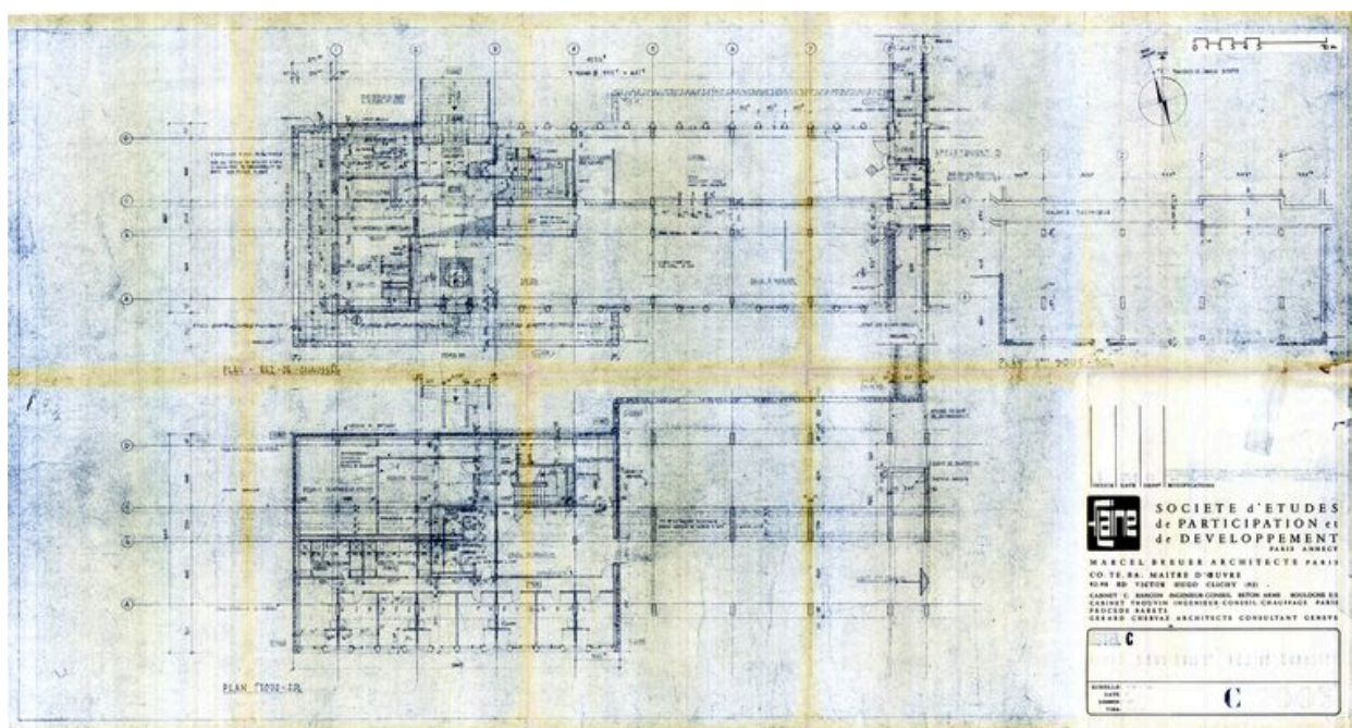
Hôtel C. Plans du sous-sol et du rez-de-chaussée. Marcel Breuer architecte, 30 octobre 1967. Modification 7 février 1968 (AC Arâches-la-Frasse)
