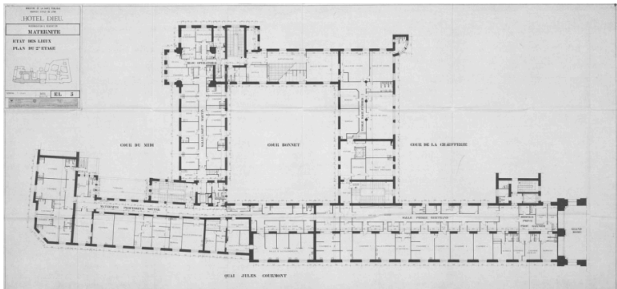
Modernisation et rénovation, maternité. Etat des lieux. Mortamet/Vidal/Manhes. SLETTI. BETSE Caillaud. Plan du 2e étage, 22 février 1978
