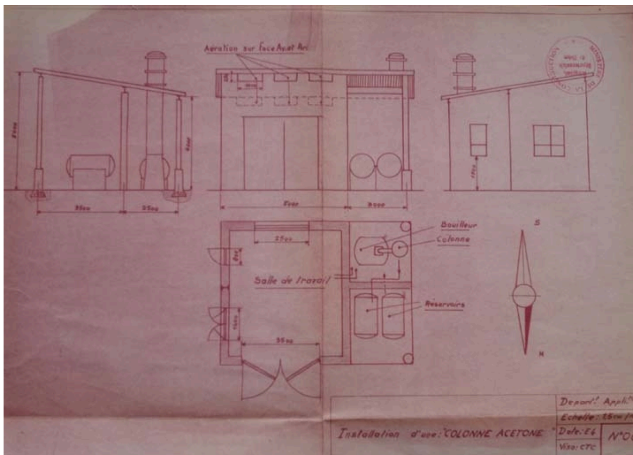
Plan du Centre Technique du Cuir ; atelier ; plan général
