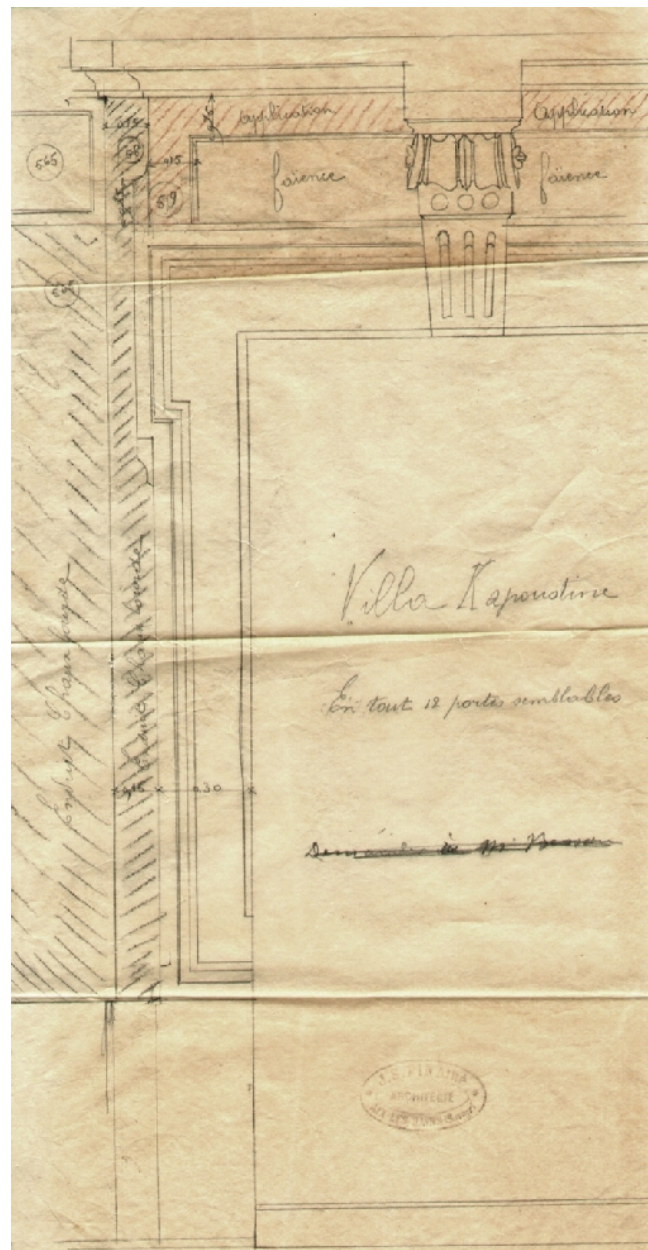
Dessin d'un encadrement de porte
