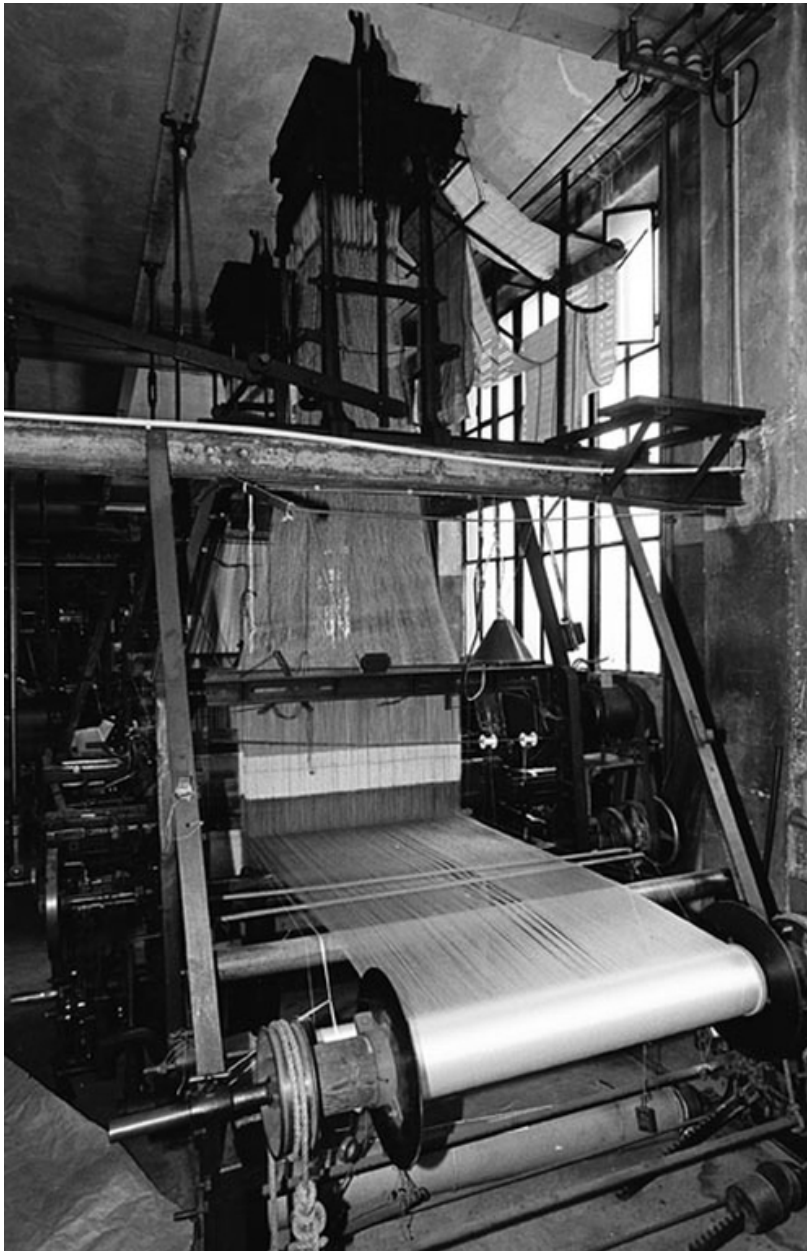
Métier à tisser jacquard n° 21, petit battant, à mécanique Verdol, de marque Diederich
