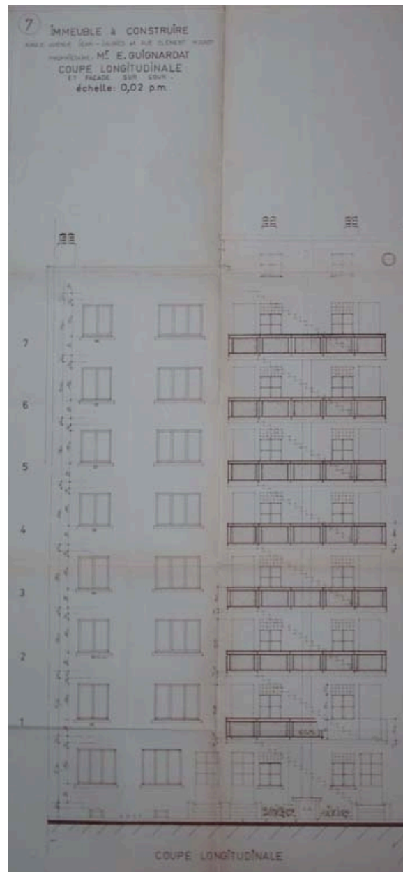
Guignardat ; construction d'un immeuble d'habitation ; façade sur cour (1956)
