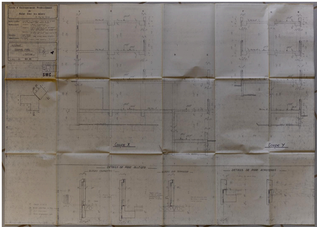
Bâtiment de l'internat. Coupes et détails (allèges, acrotères). (Archives du lycée Desaix de Saint-Eloy-les-Mines. Dossier de plans "Internat", 1981-1982. Par SMC Barrat, 5.10.1982, éch. 1/25, 123 cm x 88 cm).
