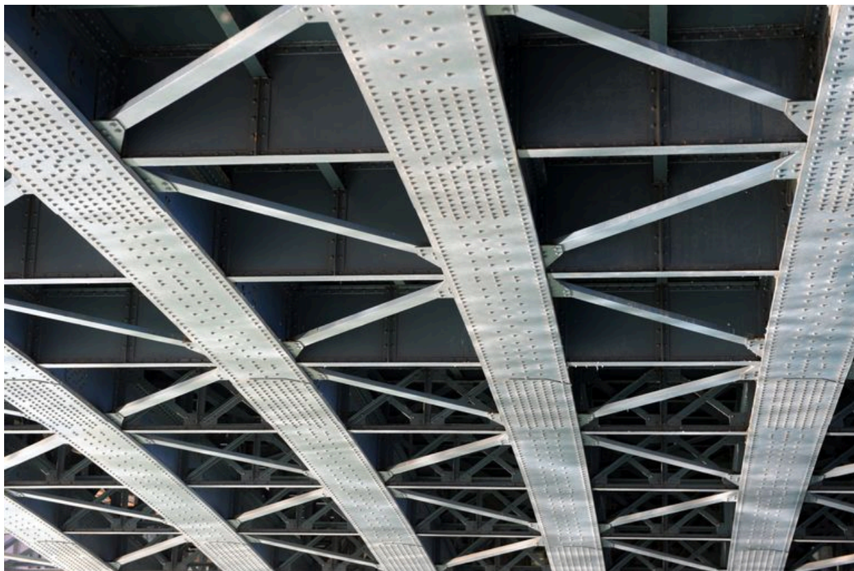
Structure de l'arche gauche, de dessous, vue de détail (depuis la rive gauche)
