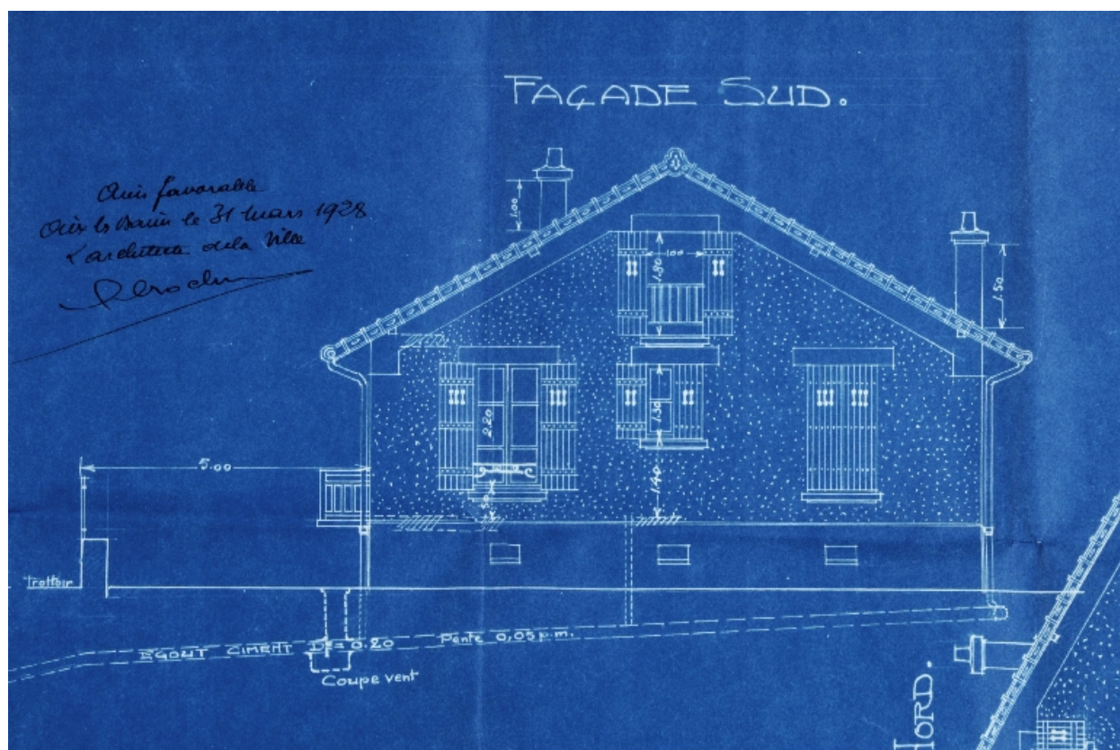
Elévation sud
