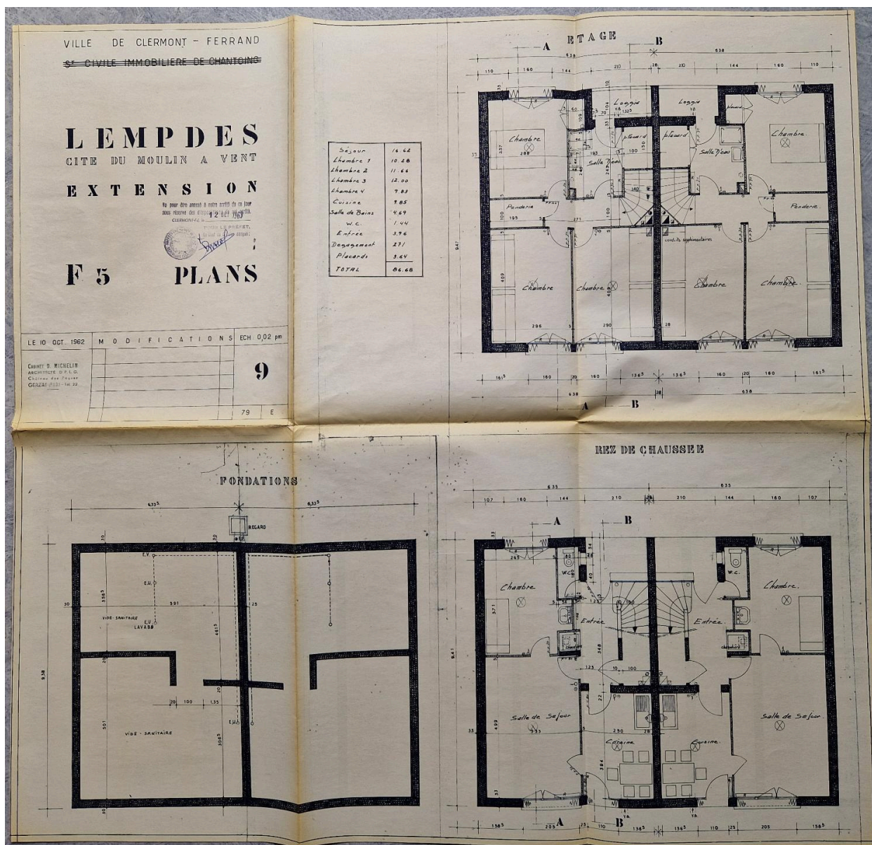
Projet d'extension de la cité de Lempdes - le Moulin-à-vent : plans des fondations, du rez-de-chaussée et de l'étage des maisons de type F5, 1962.
