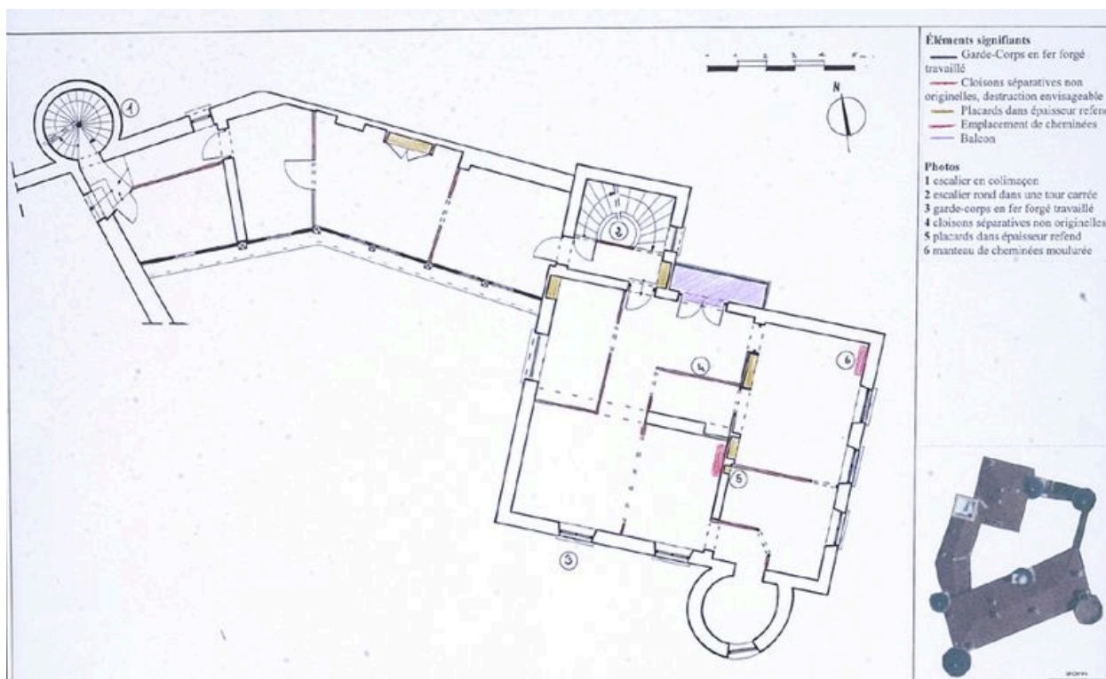
Plan du niveau 2, section nord-est, éléments significatifs
