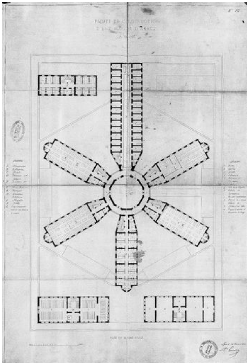
Projet de construction d'une maison d'arrêt à Lyon : plan du second étage, A. Louvier, 1860. 82 x 56,5 AD, Rhône. 1 Y 282
