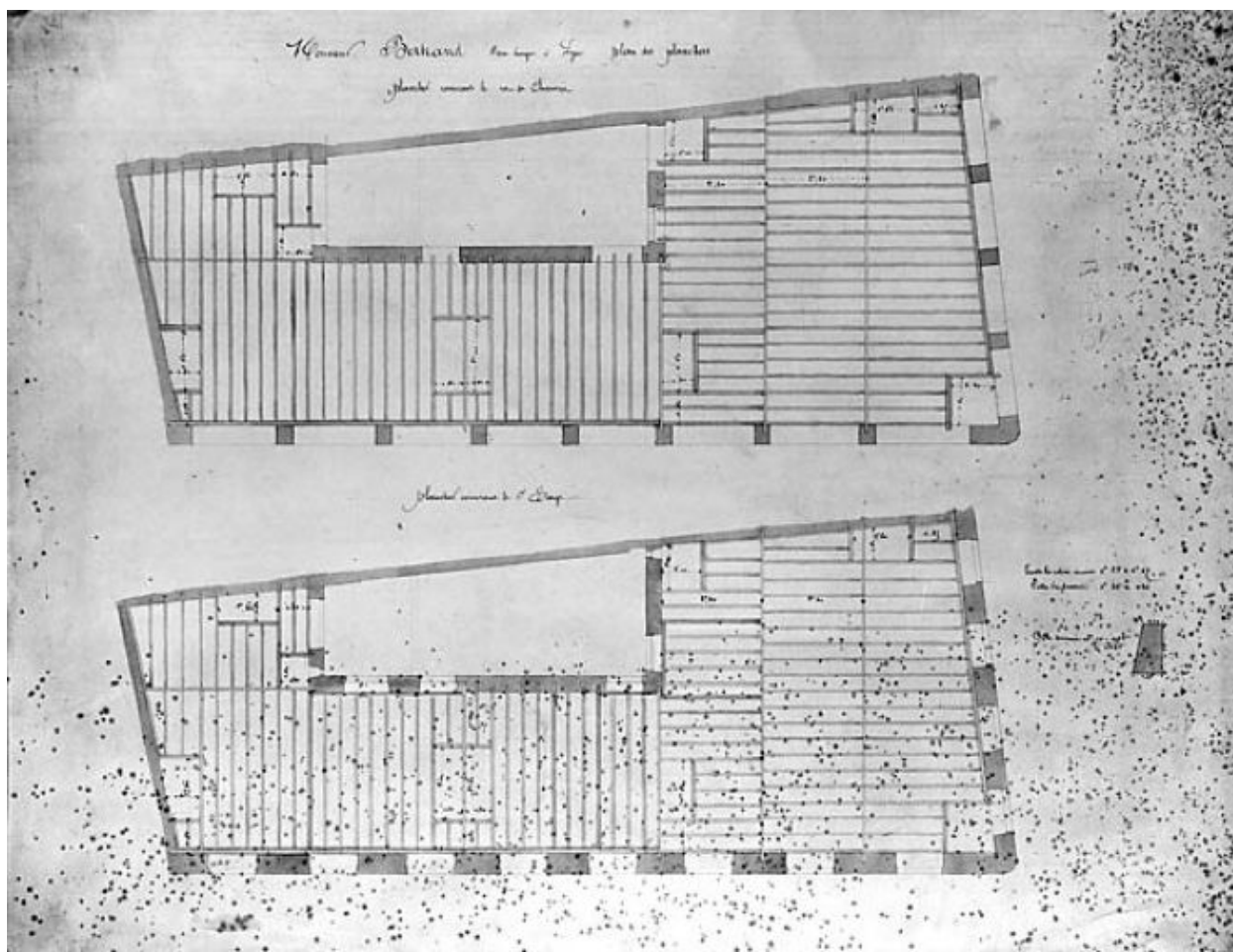
Feuille 14, Plan des planchers. Plancher couvrant le rez-de-chaussée. Plancher couvrant le 1er étage, par H. Feuga, 1869
