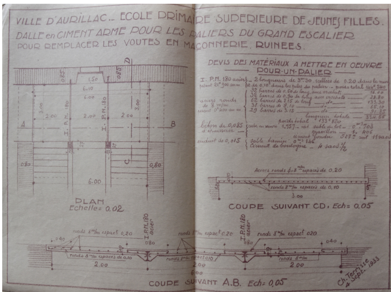
Plan et coupes pour remplacement de voûtes sur le grand escalier par Ch. Terrisse, 1933 (AD Cantal, E DEP 1500/1487)
