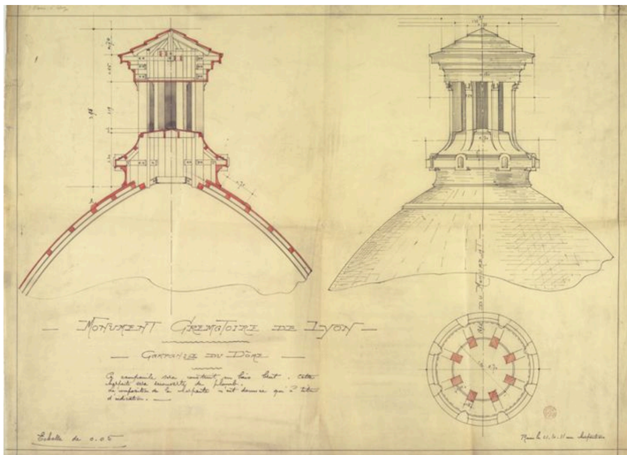
Campanile du dôme : plan, coupe, élévation
