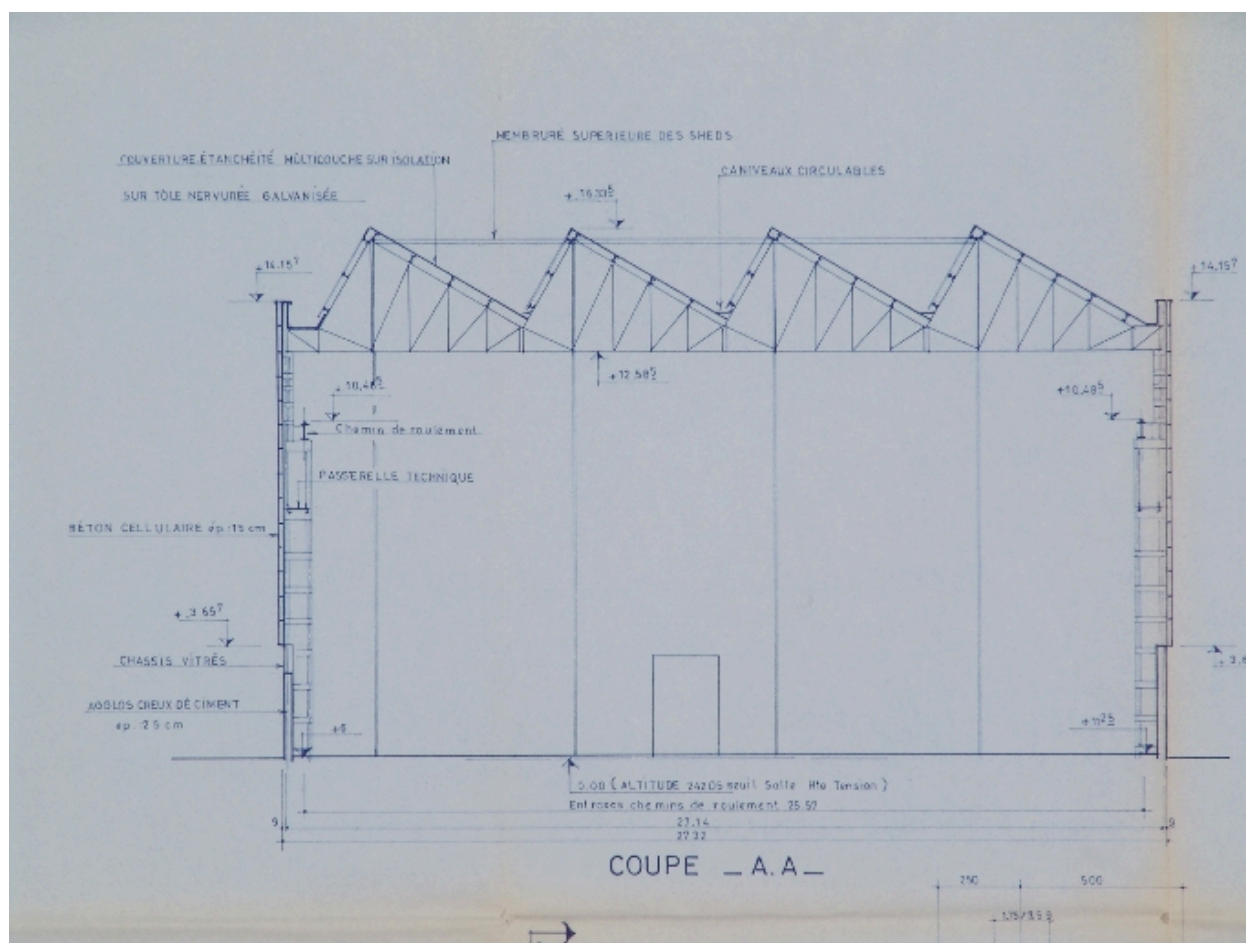
Coupe transversale de la partie ouest de la halle RM1
