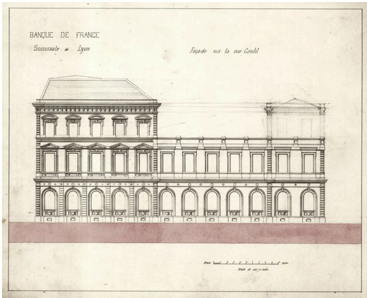
Élévation antérieure sur la rue Gentil (1855) (Banque de France, service du Patrimoine Historique et Artistique, non coté, dessin de Gabriel Crétin).
