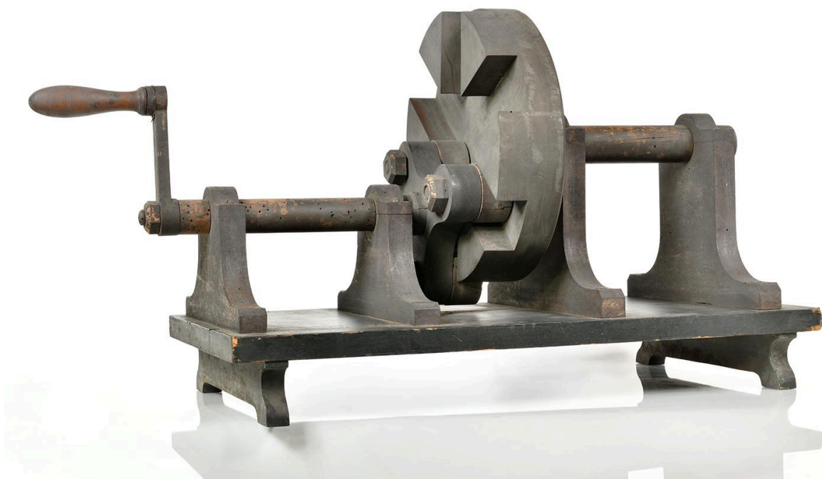
Engrenage à cônes, vue 1
