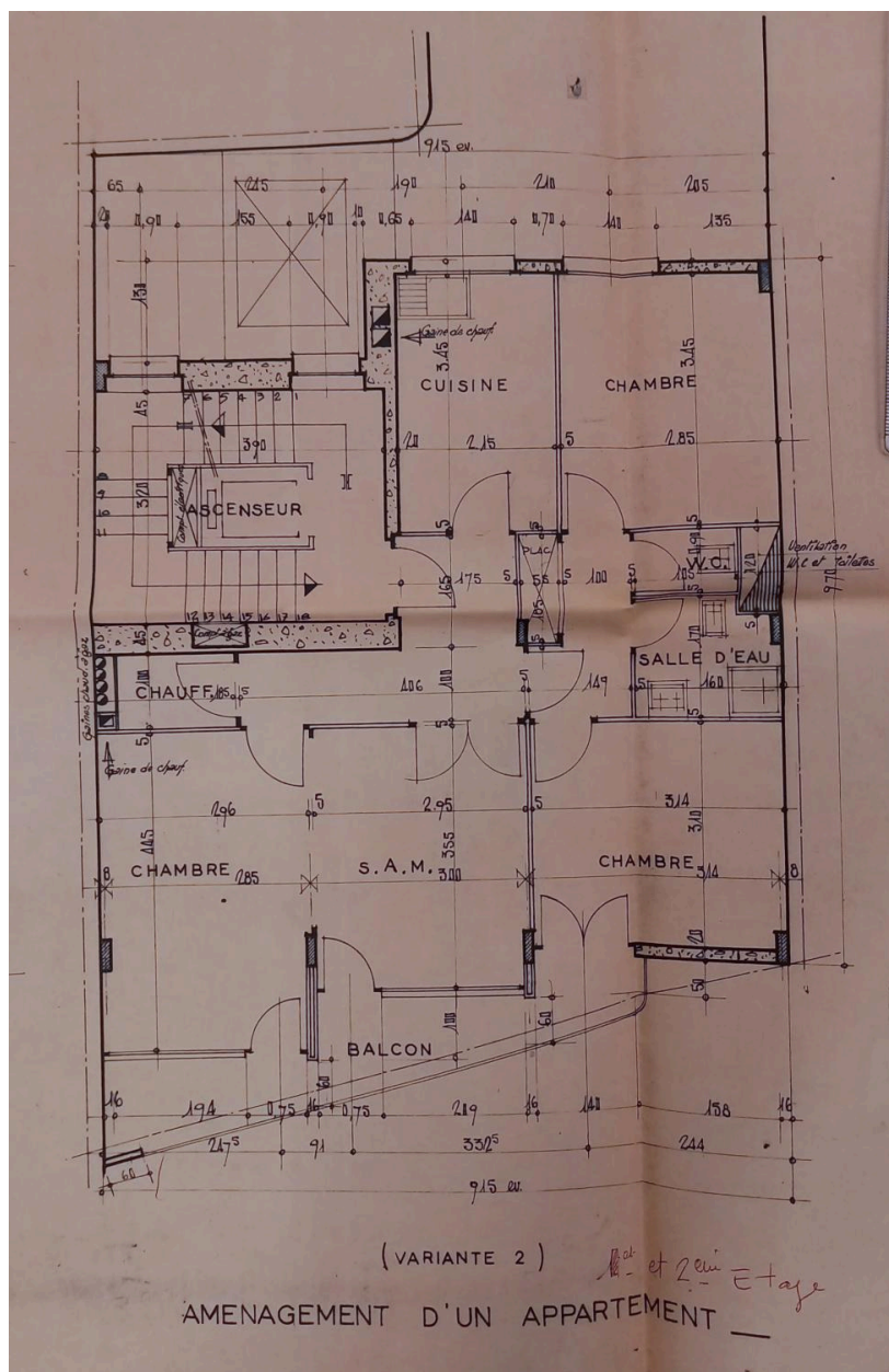
Plan des premiers et deuxième étages, 29 avenue d'Italie
