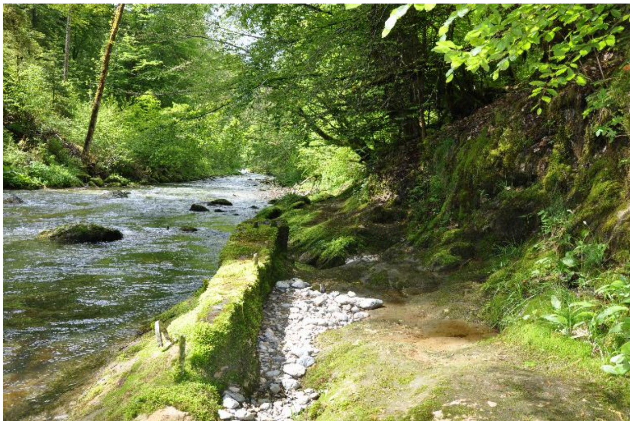
Vue de la prise d'eau.
