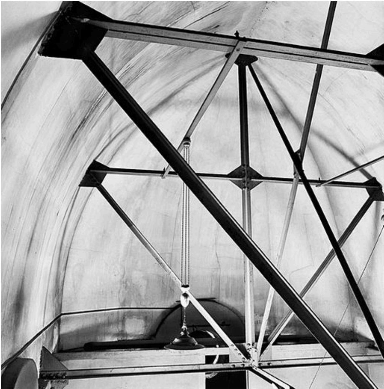
Charpente métallique boulonnée du dôme
