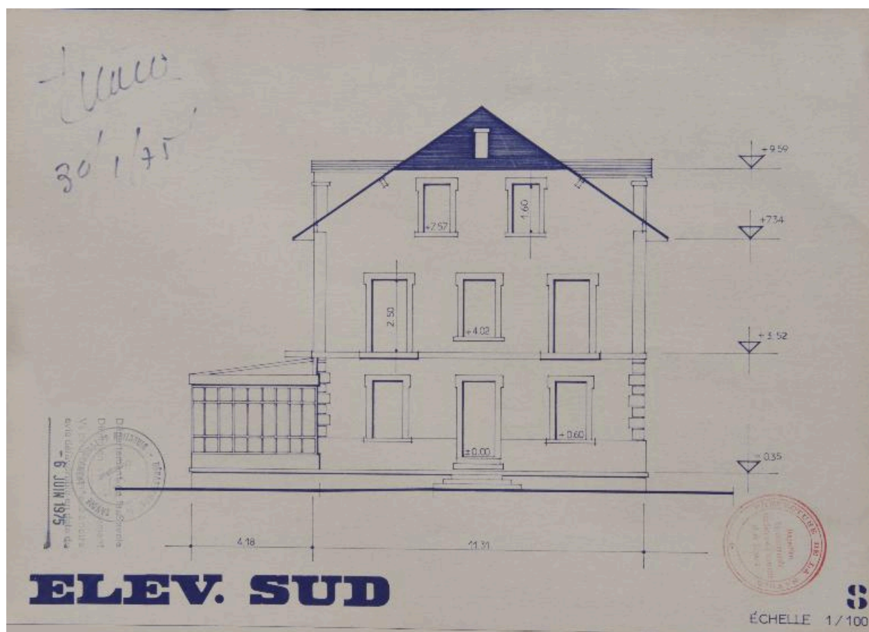
Elévation sud, 1975
