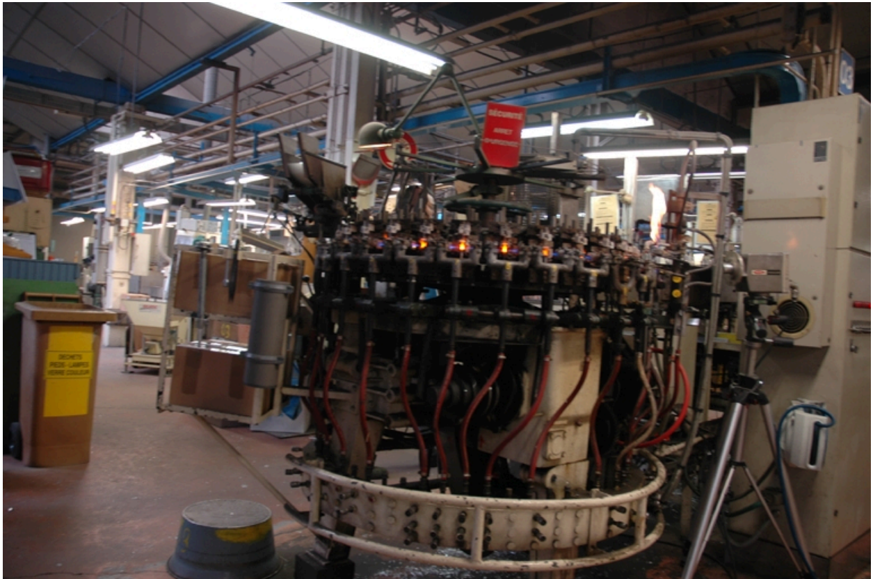
Vue d'ensemble machine filament
