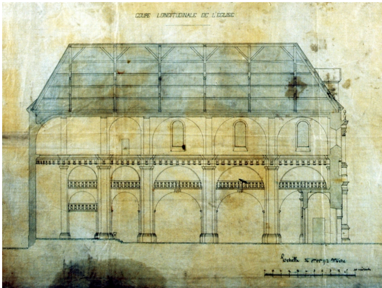
Élévations et coupes : détail n°2, par Louis Besset, 20 mars 1861 (AP Archi-consult SARL)
