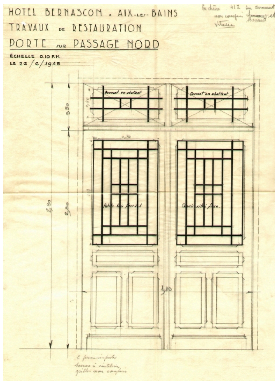
Elévation de la porte sur passage nord
