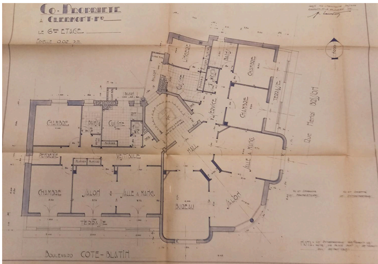
Plan d'un étage. Comparaison n°76 bd Cote-Blatin (projet non réalisé)
