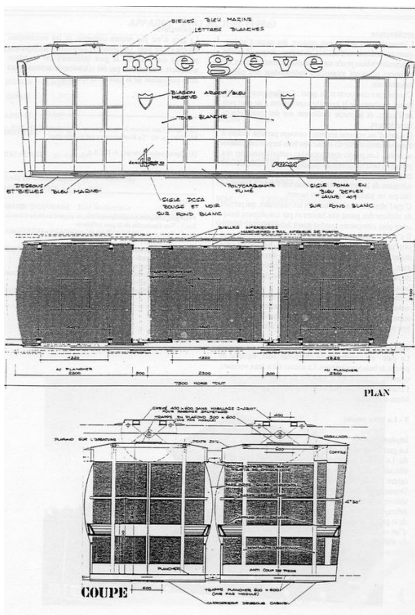
Téléphérique de Rocharbois. Plan, coupe, élévation des cabines / [Yann Misson, 1985]
