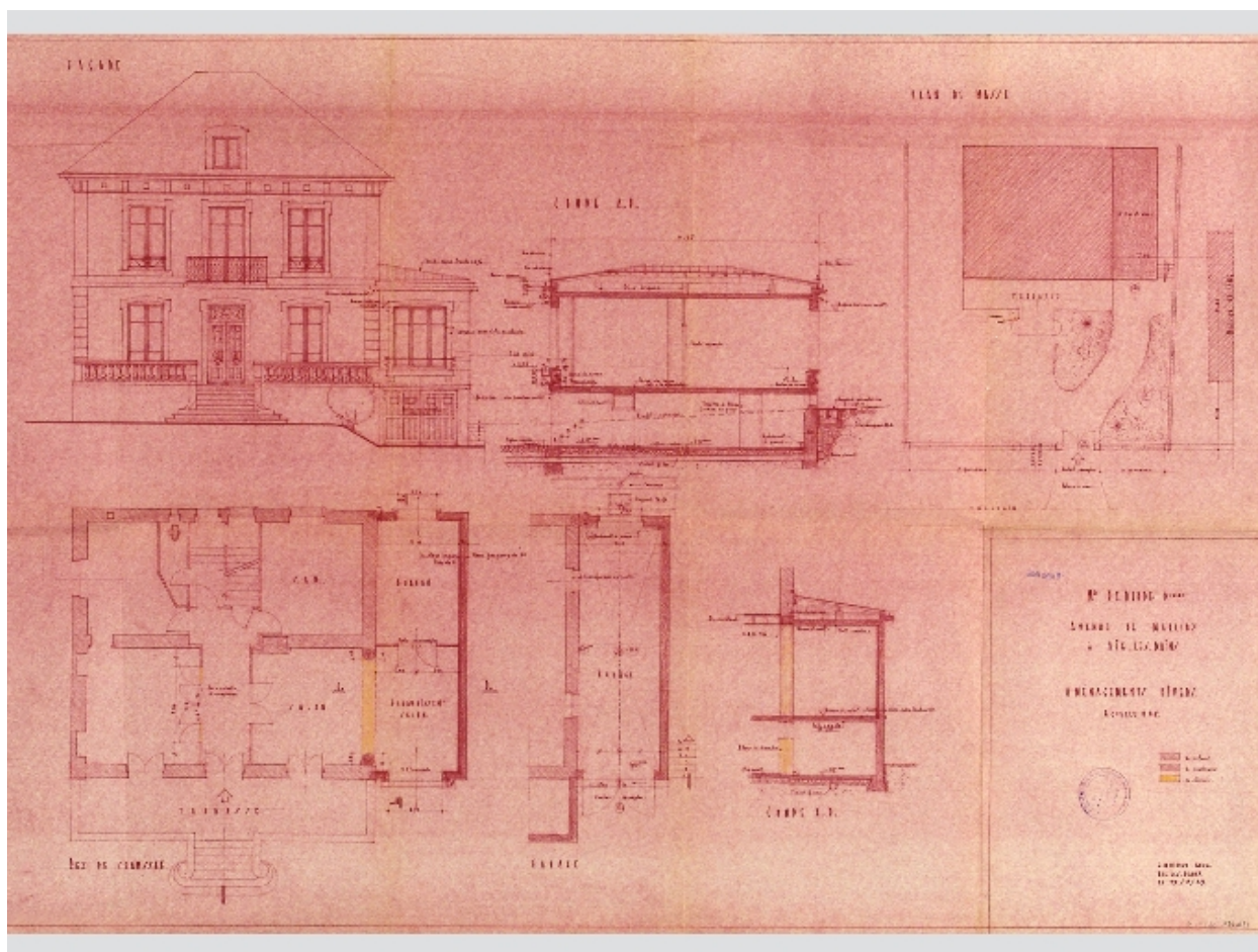
Plans, coupes et élévation principale
