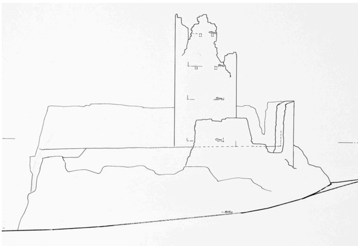
Commune d'Ecotay-L'Olme (Loire). Restauration du château. Façades. Vue nord (1).
