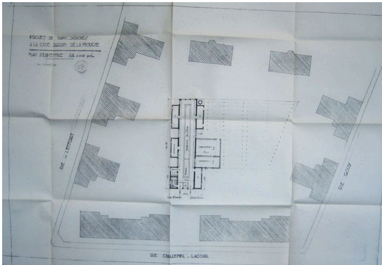
Plan d'ensemble. Projet de bains douches lavoir au centre de la cité jardin de la Mouche. A. E. Chollat et t V. Robert architectes, 11 avril 1930. Echelle 1 : 200 (Arch. mun. Lyon)
