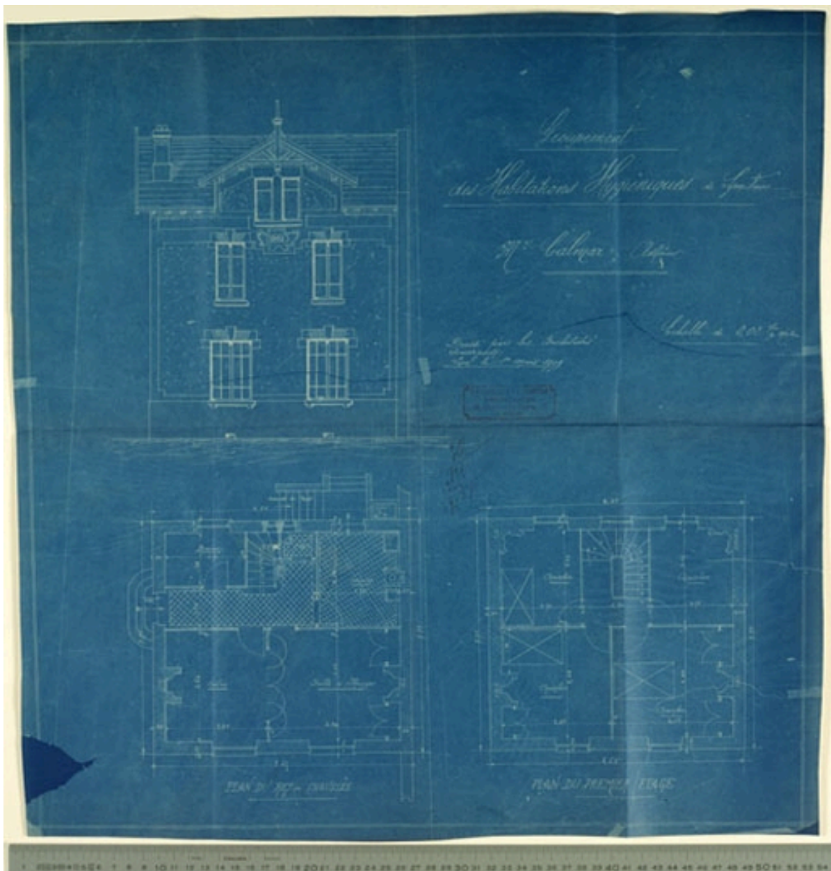
314 WP 62, 1909 permis 288, plans, façade d'une maison individuelle au 18 rue Littré
