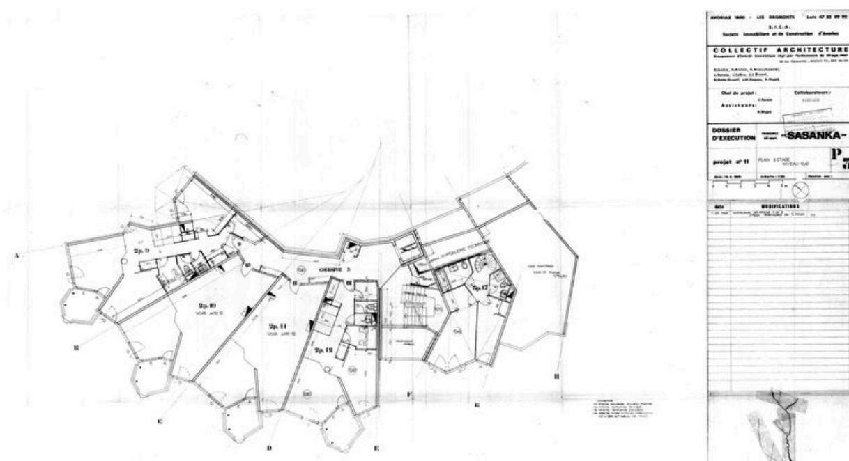
Dossier d'exécution / Collectif Architecture, 15 juin 1969. Plan du 3e étage (AC Morzine)
