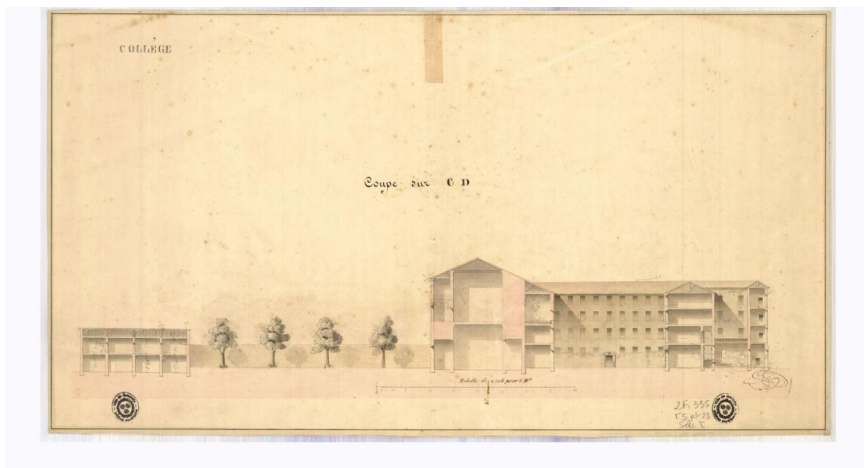
Collège royal, état des lieux : coupe transversale, 1837 (AC Grenoble, 2 Fi 335)
