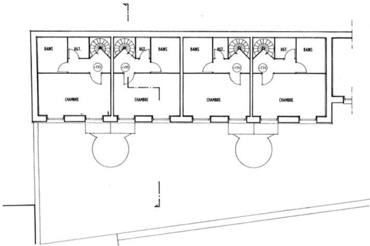
Plan de l'étage du corps de bâtiment sud / B. Verrier, I. Gaillard, 7 juin 1990. Ech. 1 : 100
