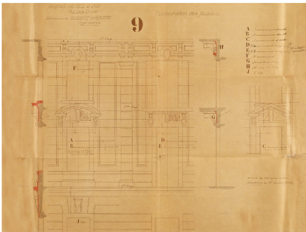
Détails d'élévation, n° 9
