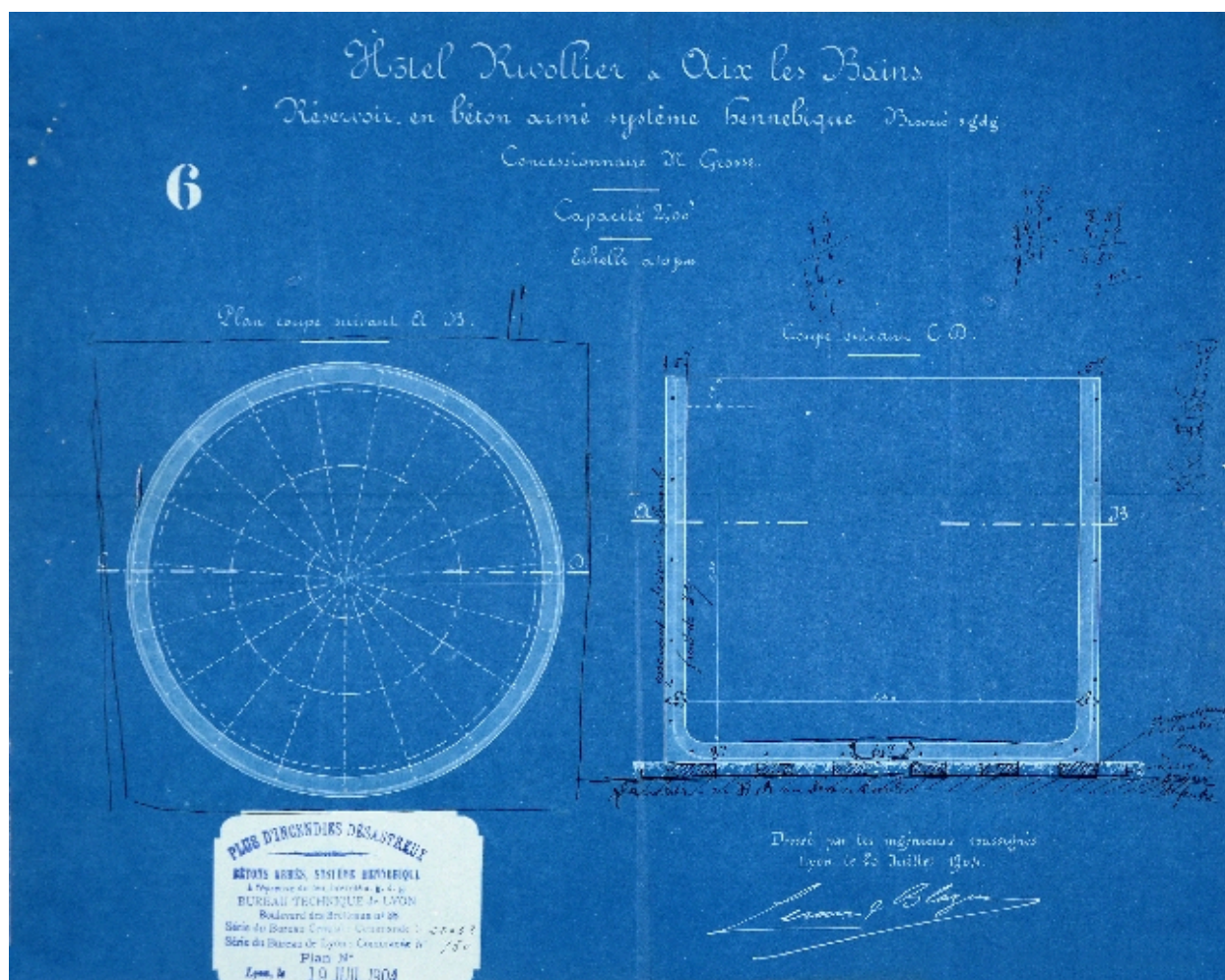
Plan et coupe du réservoir
