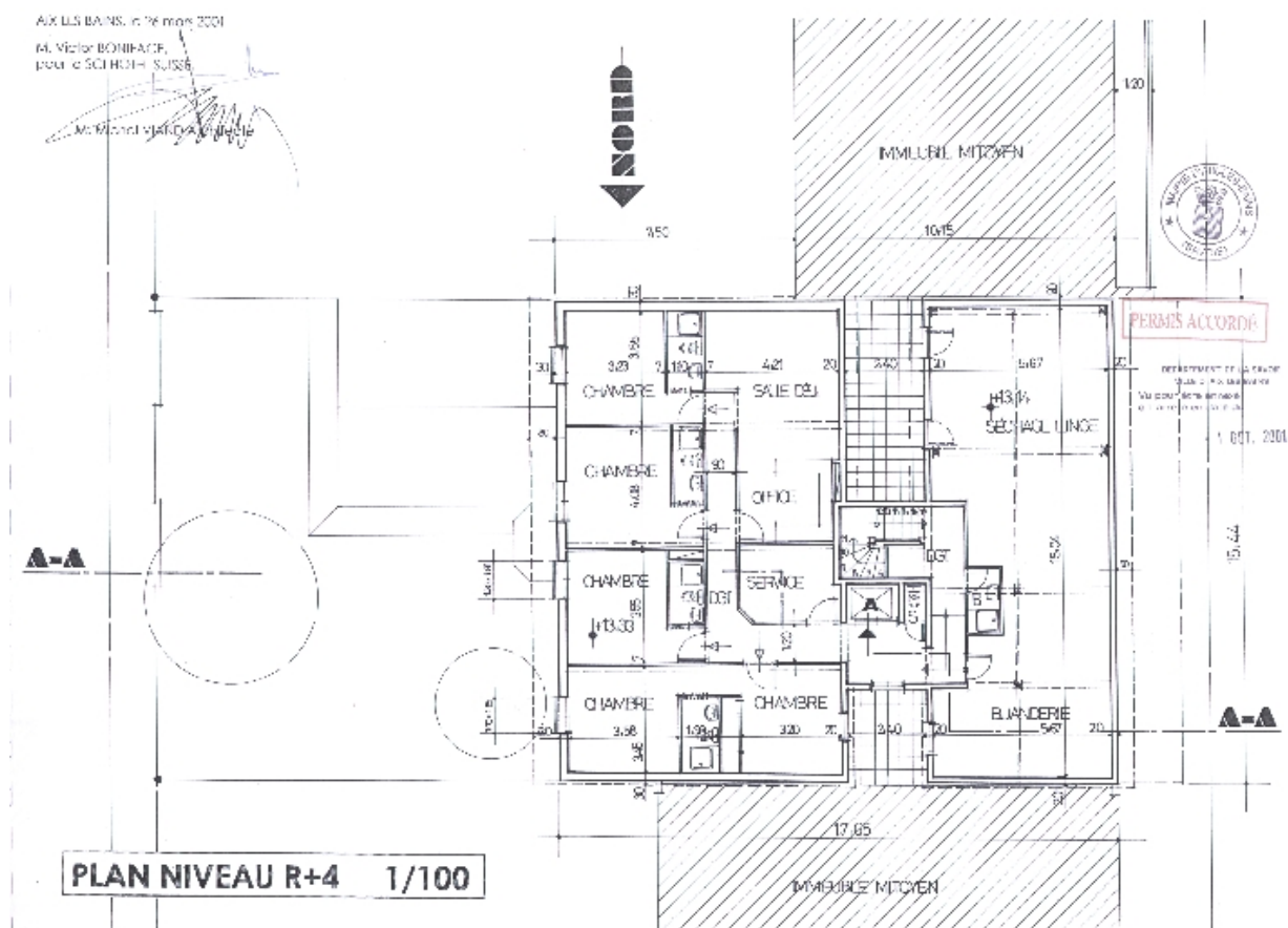
Plan du quatrième étage avant transformation
