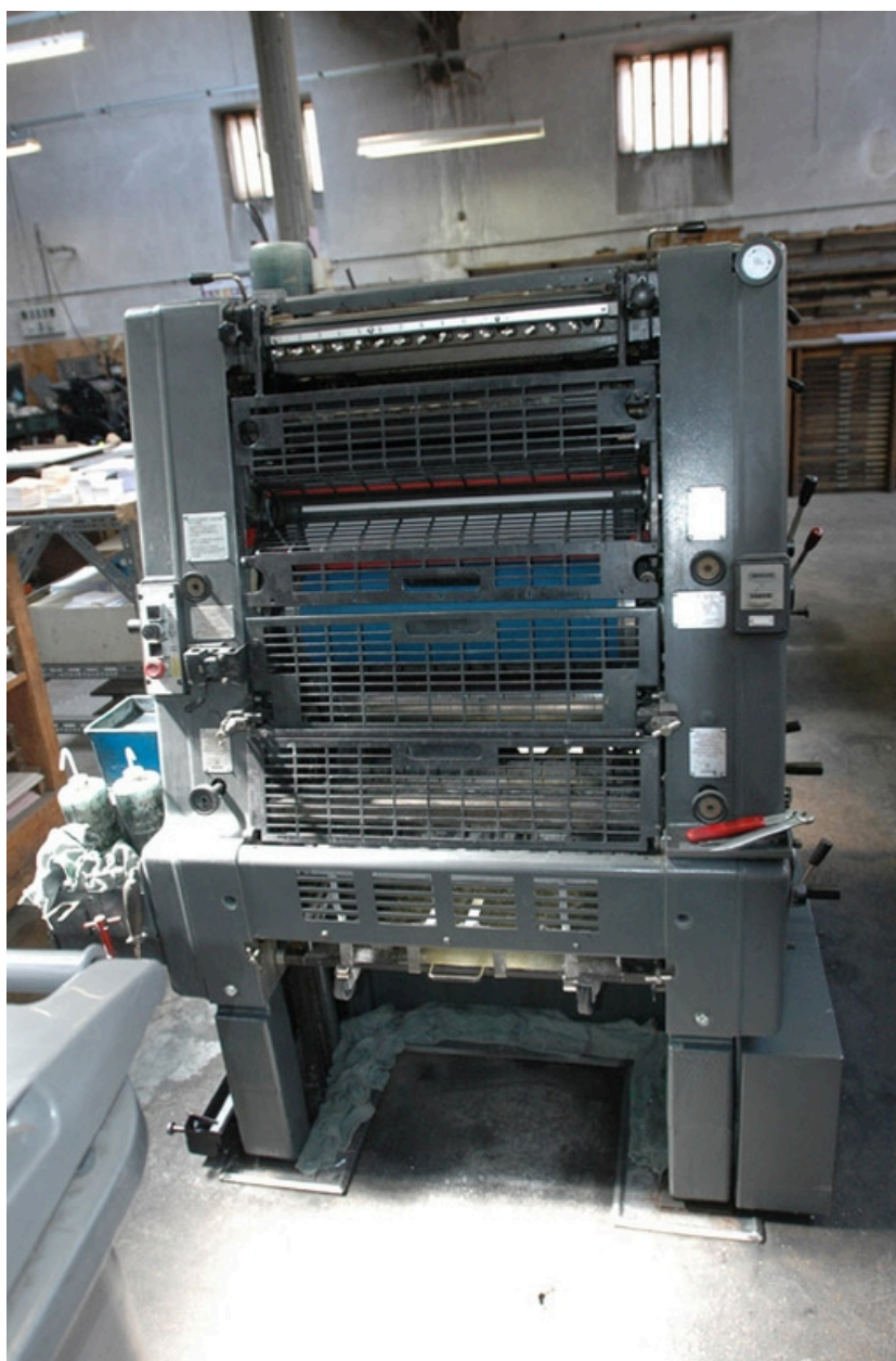
Machine offset monochrome, vue arrière, (cf n° 4 sur la plan).
