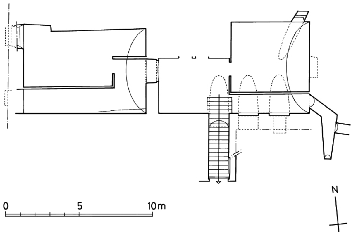
Plan partiel du sous-sol, relevé expédié et schématique.
