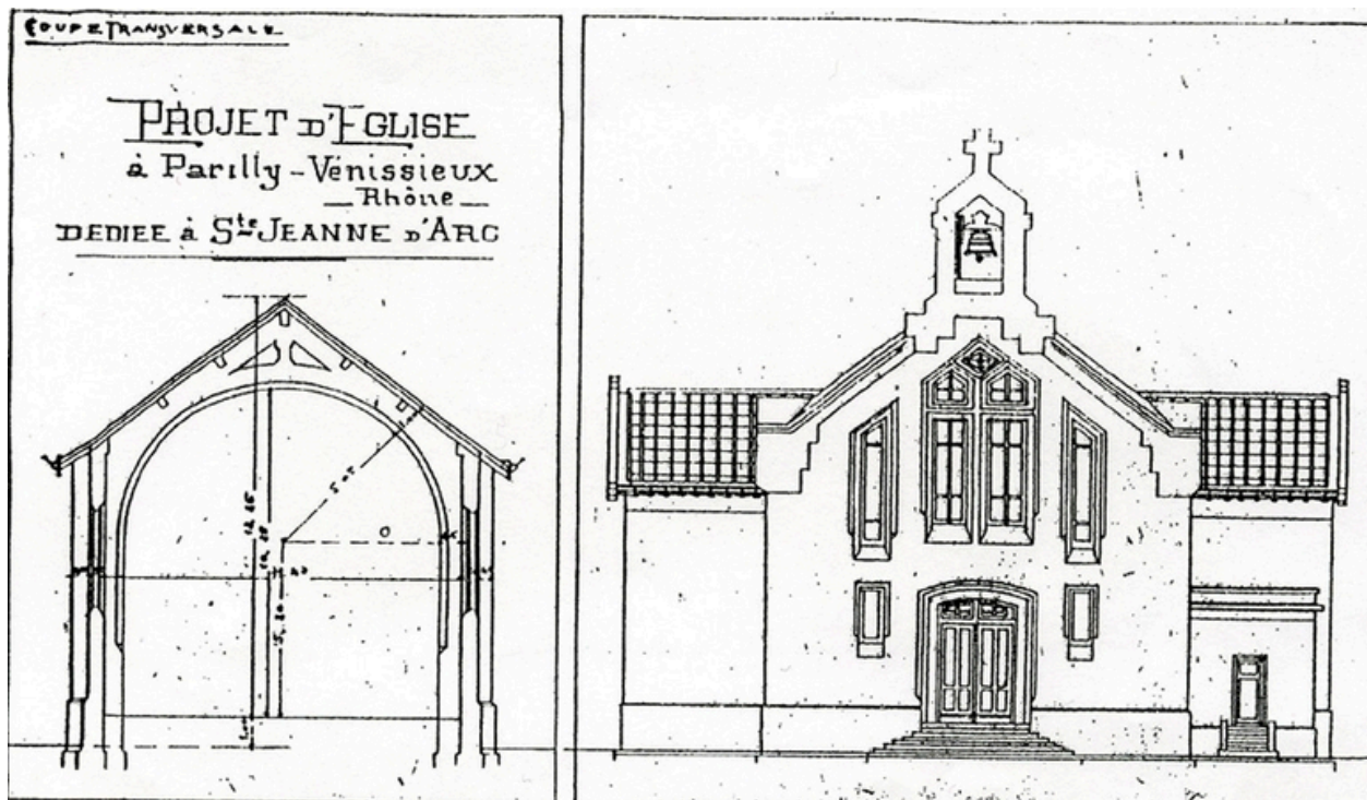
Coupe transversale : projet de l'église à Parilly-Vénissieux.
