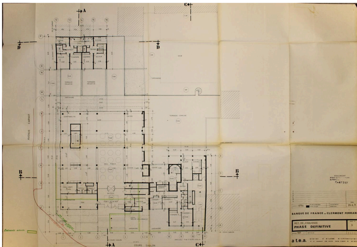
Clermont-Ferrand, succursale de la Banque de France, plan du rez-de-chaussée, 1971, agence ATEA Lagneau-Weil-Dimitrijevic (Archives municipales de Clermont-Ferrand, 2001 W 296).
