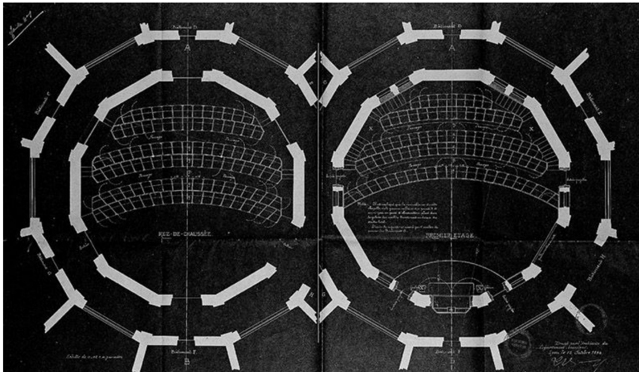
Transformation de la maison d'arrêt et de justice de Lyon en prison cellulaire : plans du rez-de-chaussée et du premier étage de la chapelle-école, 1894. 12 octobre 1894, 48 x 84 AD, Rhône. 1 Y 283
