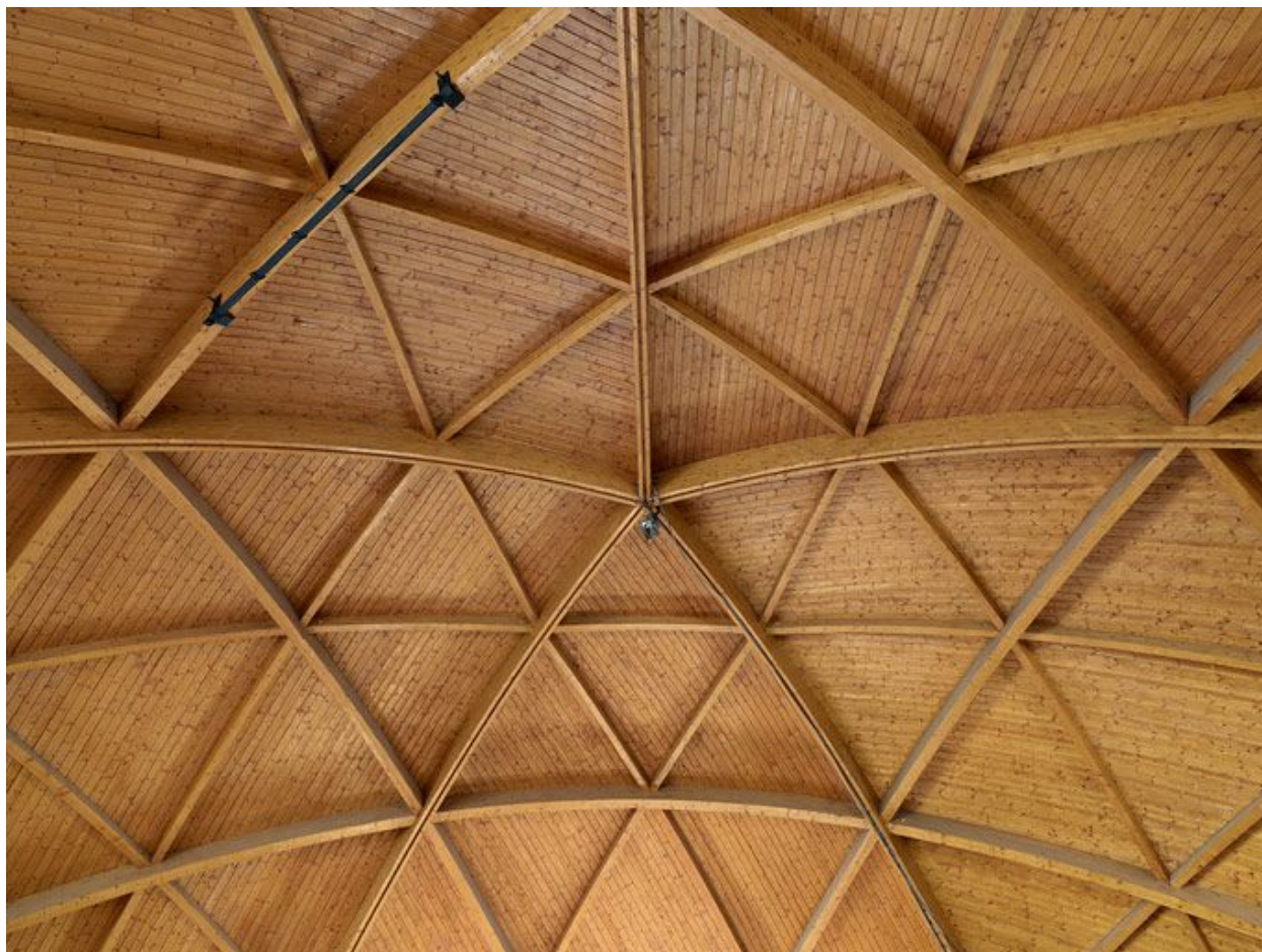
Auditorium. Détail de la charpente. Dessin à l'origine du logo des Arcs
