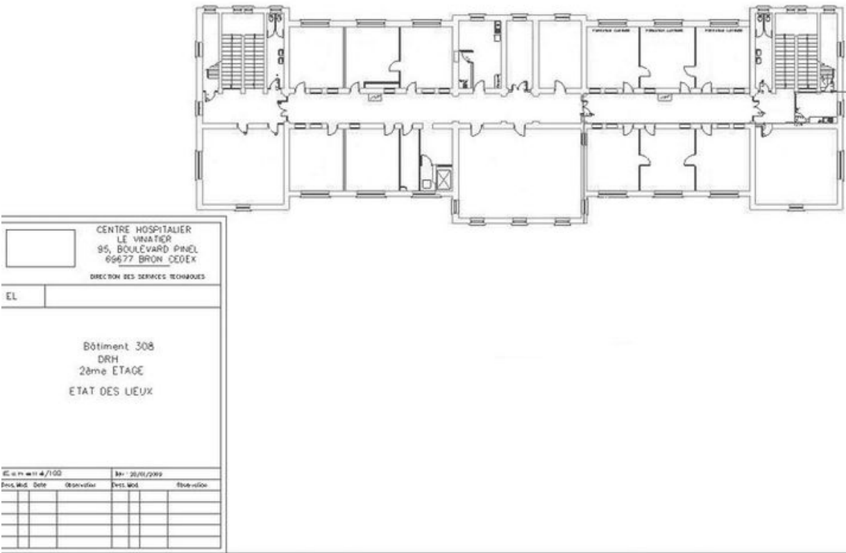
Plan du 2e étage. Les éléments en gris sont des adjonctions
